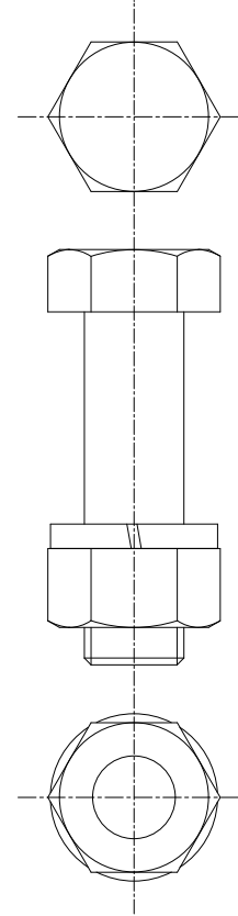
ワッシャー無 スプリング付
